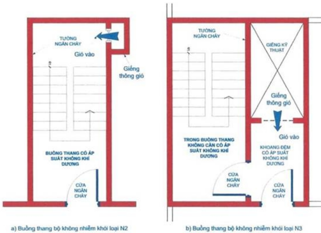
Hình I.9 - Minh họa buồng thang bộ không nhiễm khói loại N2 và N3
